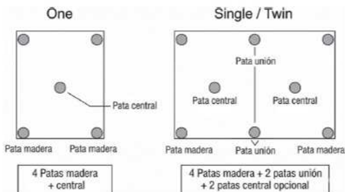
Configuración de patas
